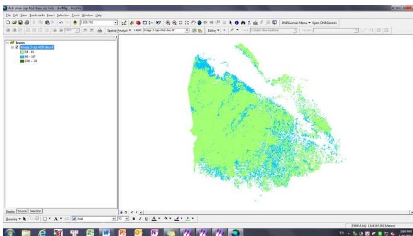
Hình 3.14: Ảnh phân 3 cấp TAGTB trong ArcGIS
