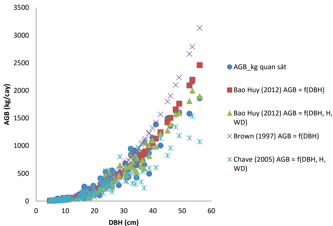
Hình 1.6: So sánh sự phù hợp của các mô hình trong đề tài với mô hình của Brown (1997) và Chave (2005)
