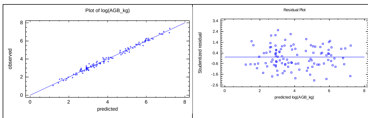
Hình 1.7: Quan hệ giá trị dự báo AGB với quan sát và biến động phần dư (residual) của mô hình 4 biến \log(\text{AGB}) = f(\log(\text{DBH}), \log(\text{H}), \log(\text{Ca}), \log(\text{WD}))
