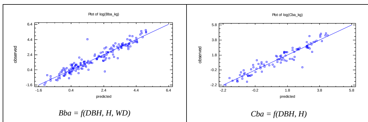
Hình 1.3: Quan hệ giữa giá trị ước lượng sinh khối và carbon tích lũy trong vỏ qua mô hình với thực tế
