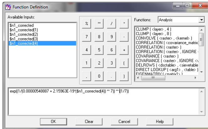
Hình 3.11: Chạy mô hình quan hệ TAGTB = f(B4) để tạo pixel ảnh theo sinh khối
