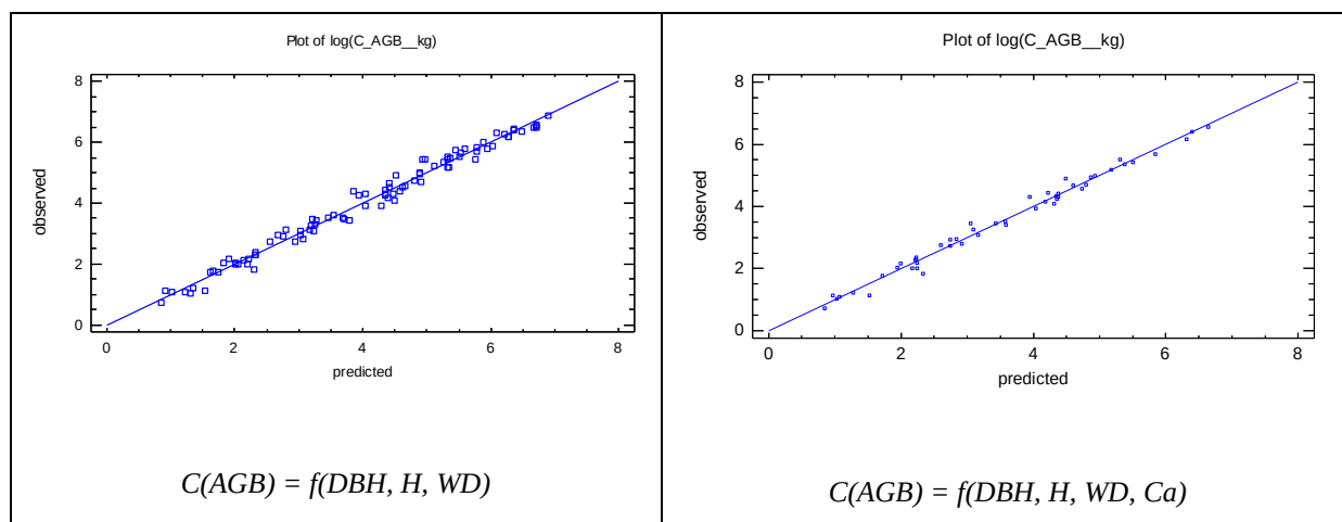
Hình 1.8: Quan hệ giá trị ước tính C(AGB) qua mô hình có biến số khác nhau với giá trị quan sát
