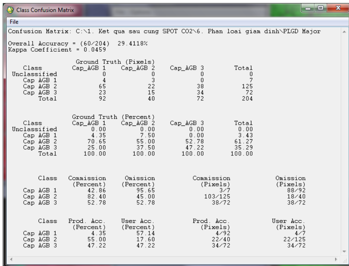
Hình 3.17: Ma trận đánh giá độ tin cậy của phân loại rừng có giám định theo sinh khối
