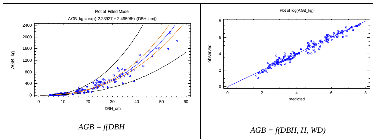
Hình 1.5: Quan hệ AGB với các biến số khác nhau
