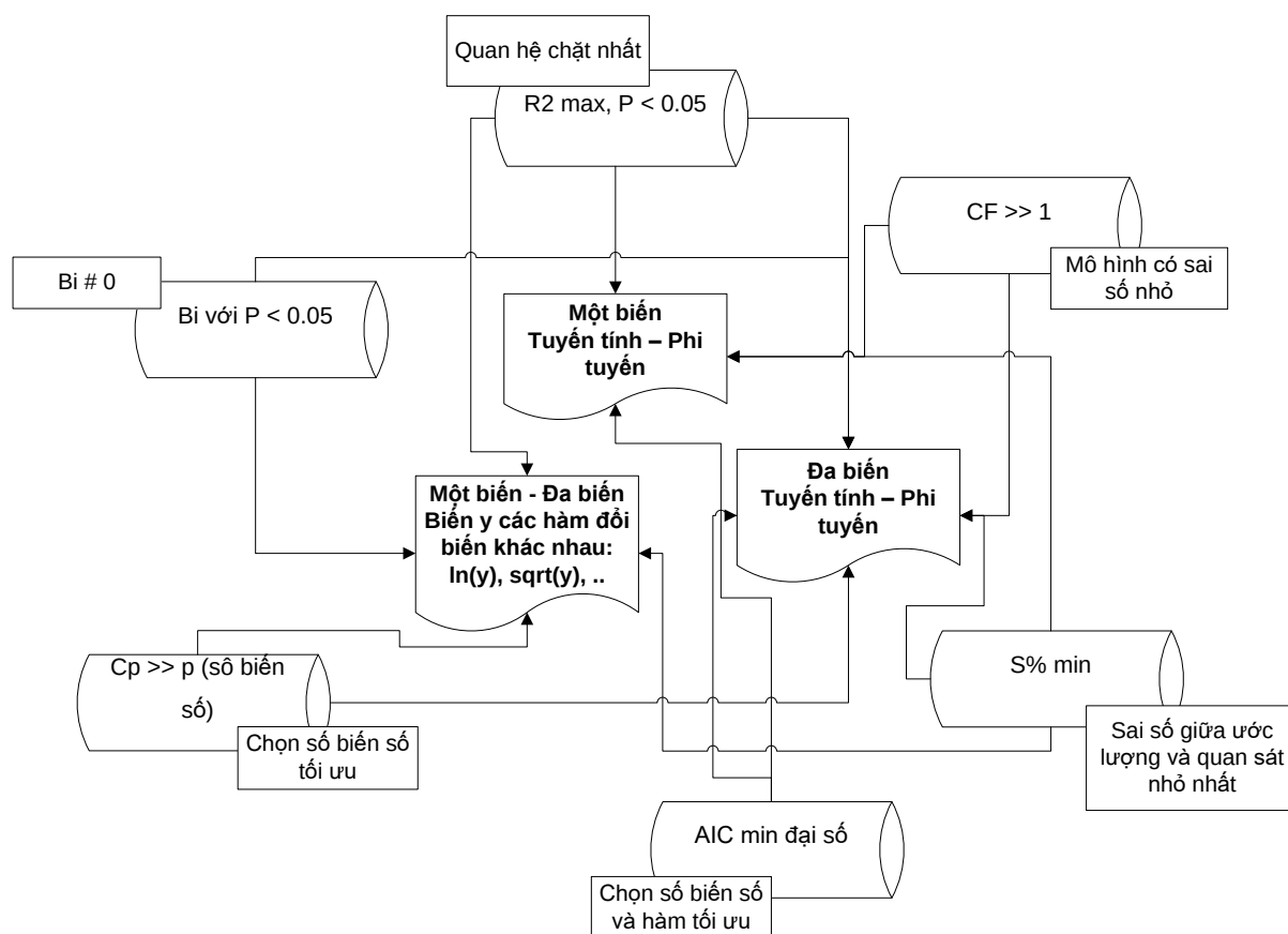
Hình 0.15: Các tiêu chuẩn thống kê để lựa chọn biến số và hàm tối ưu
