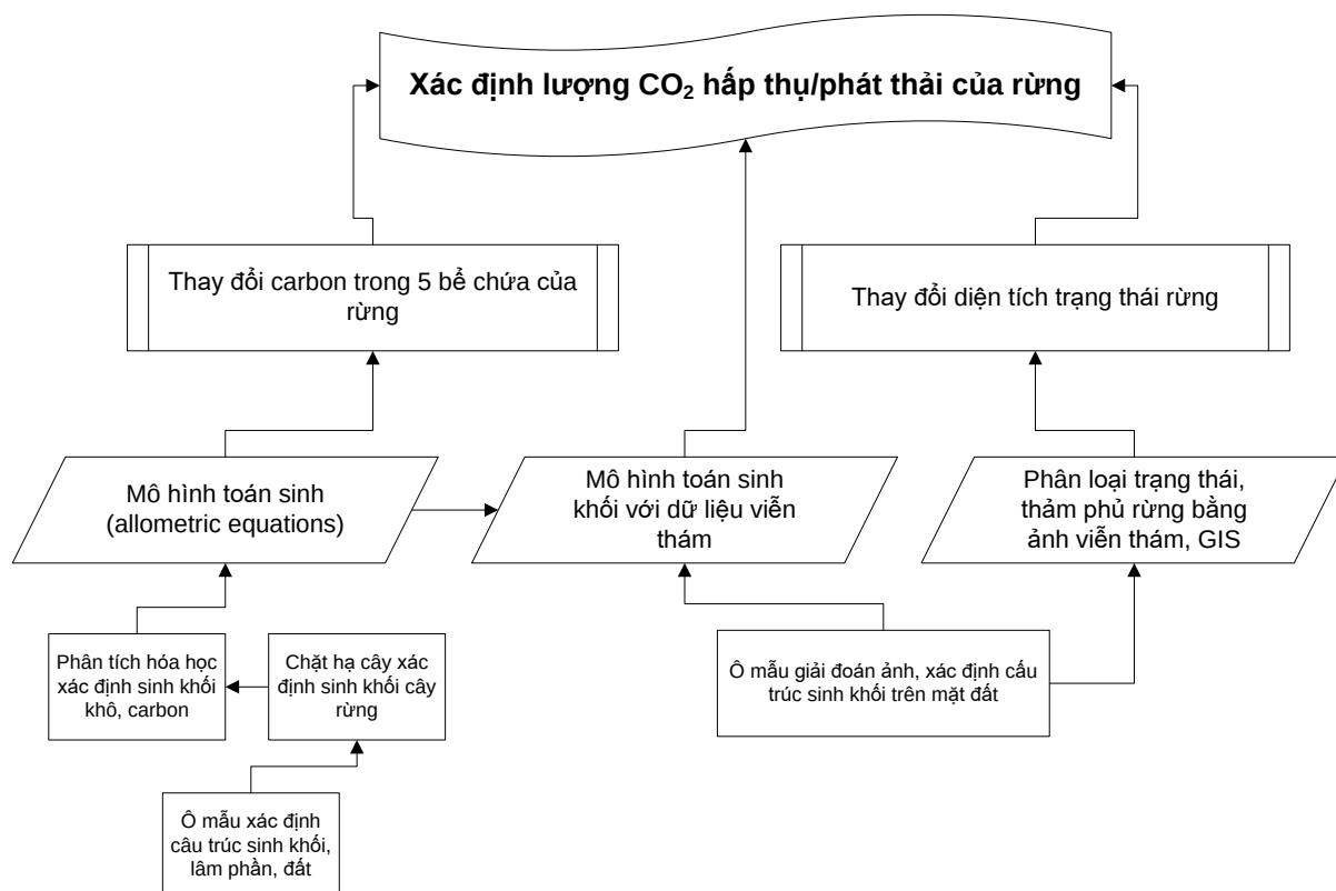
Hình 0.3: Sơ đồ tiếp cận nghiên cứu
