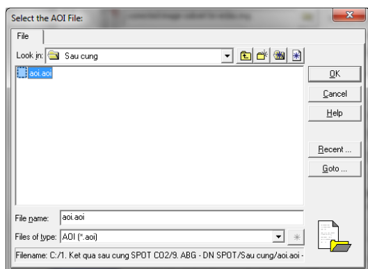
Hình 3.10: Lập mô hình tạo ảnh sinh khối rừng Erdas
