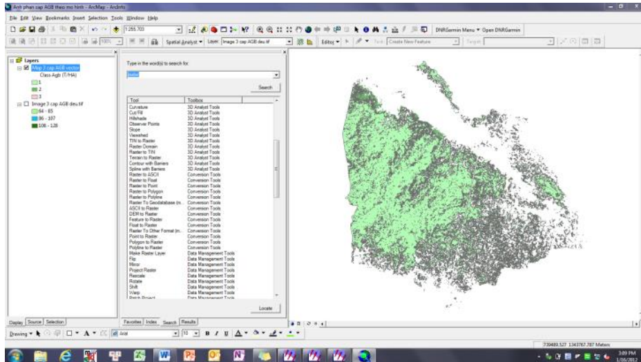
Hình 3.15: Bản đồ vector 3 cấp sinh khối rừng trên mặt đất
