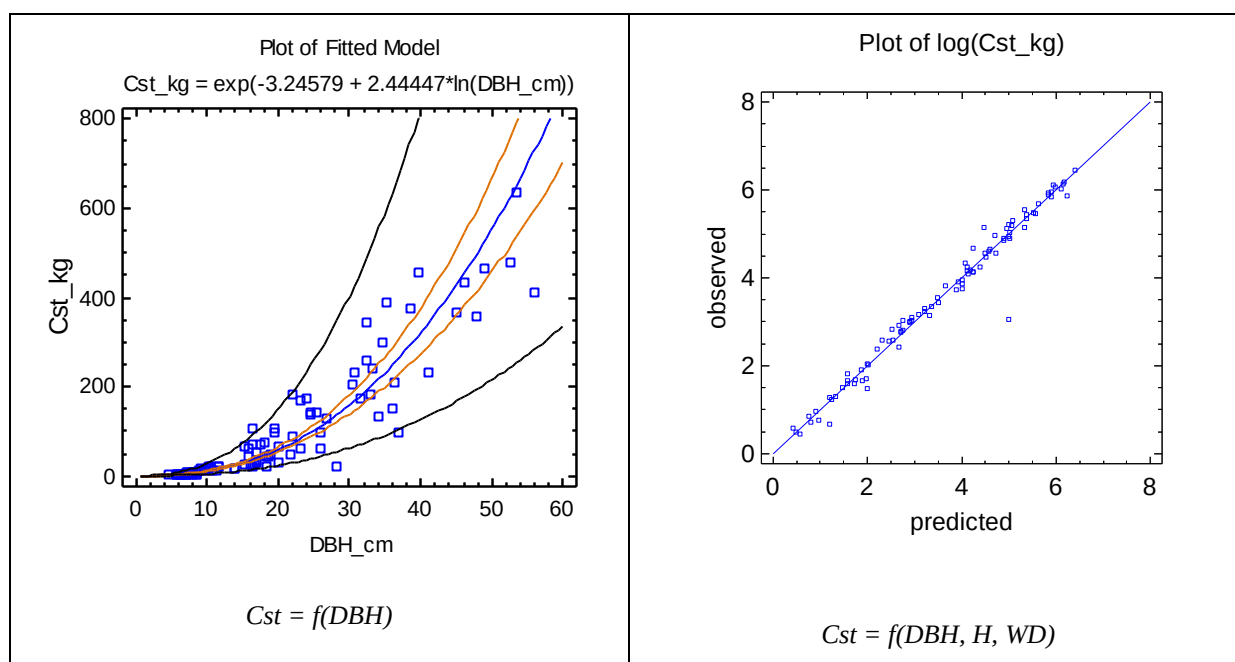
Hình 1.2: Quan hệ giá trị dự báo Cst với quan sát theo mô hình 3 biến DBH, H và WD hoặc chỉ với DBH
