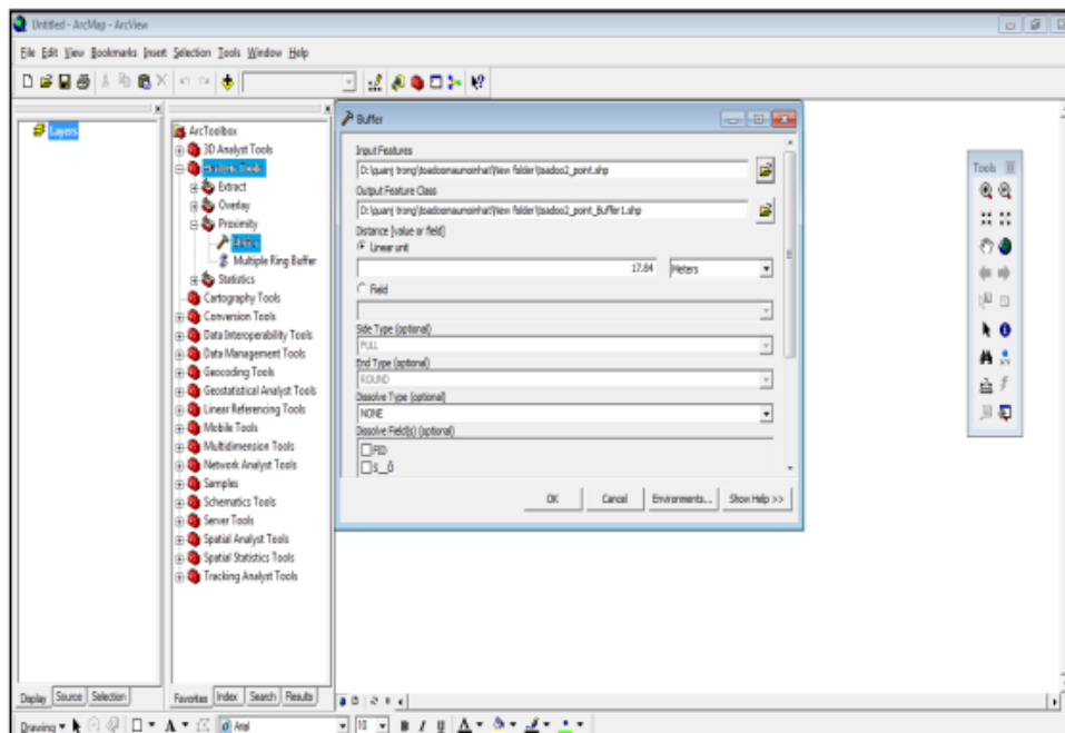
Hình 3.7: Tạo vùng đệm buffer cho ô mẫu trên phần mềm ArcGIS
