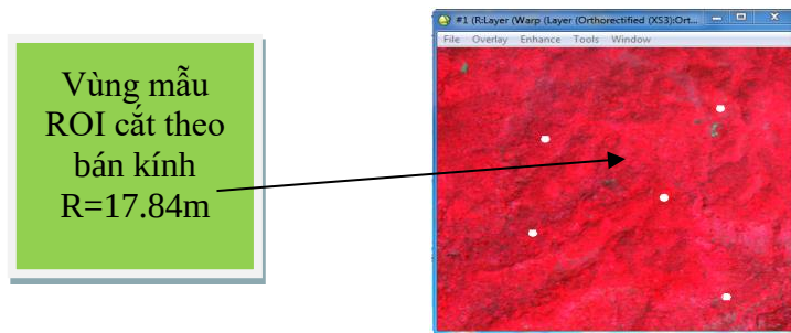
Hình 3.8: Chồng các ô mẫu lên ảnh với bán kính 17.84m
